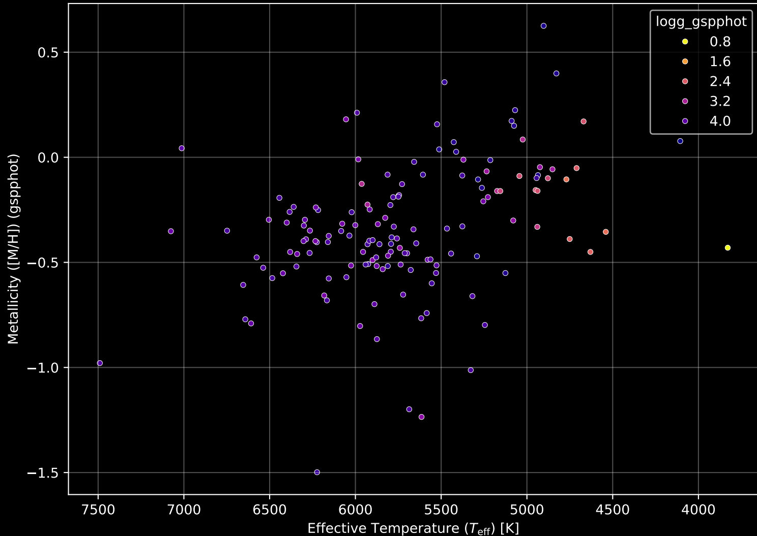
GALAH DR4 Field: [7242] Stellar Population Parameters (n= 144)
